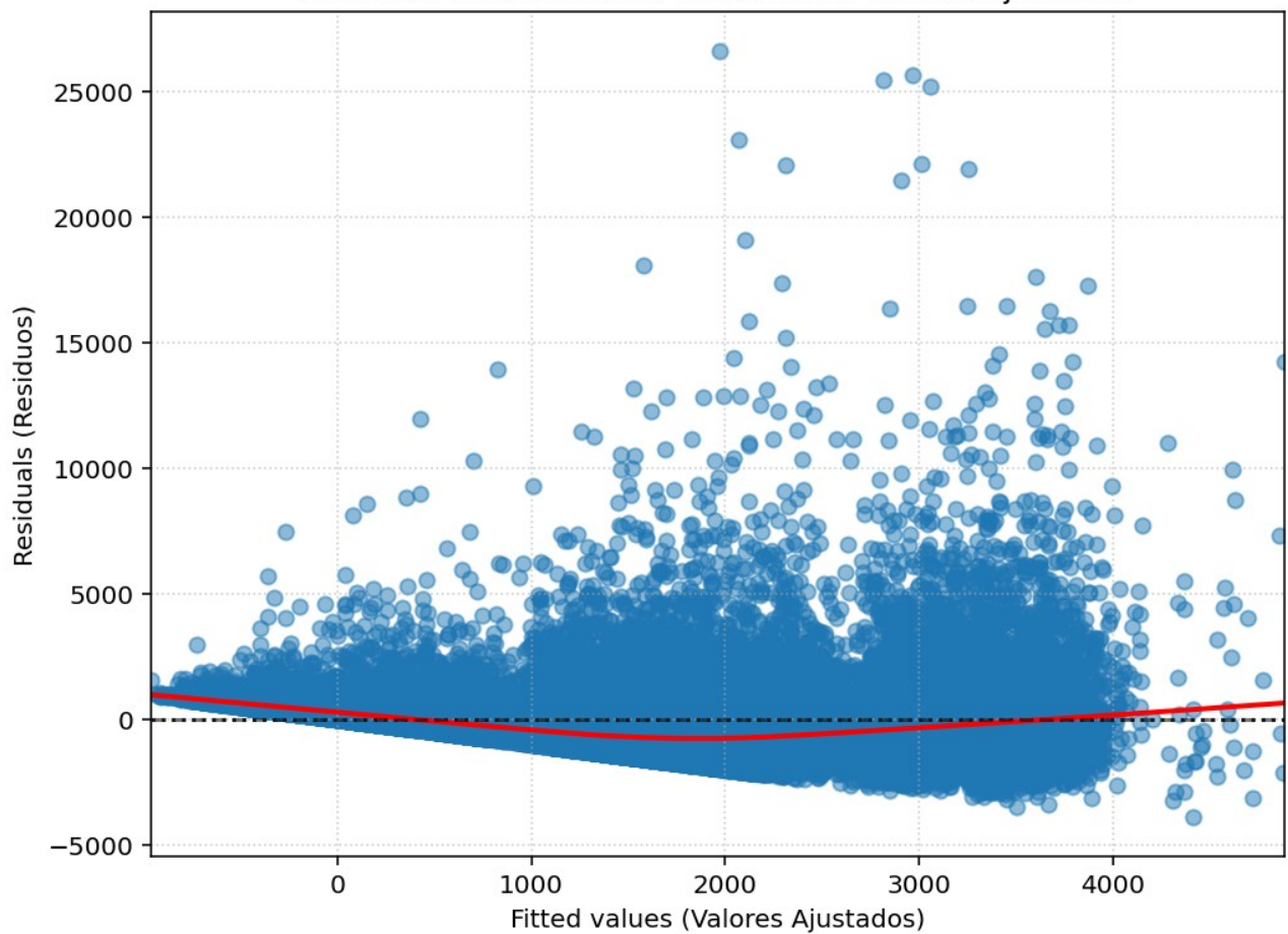
Asunción de Linealidad: Residuos vs Valores Ajustados
