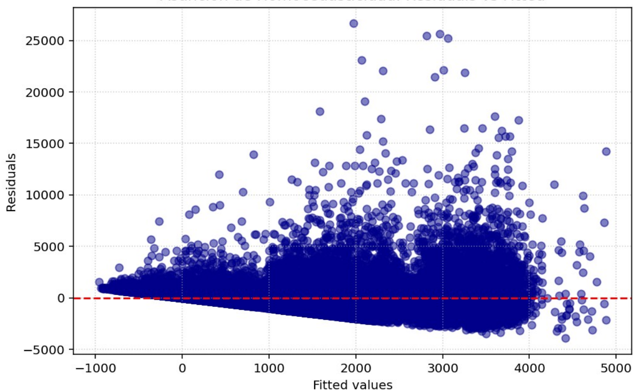
Asunción de Homocedasticidad: Residuals vs Fitted
